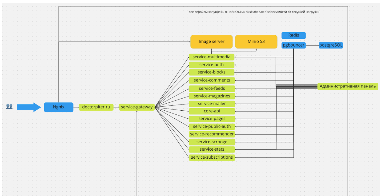
Рис. 1. Общая схема ПО
